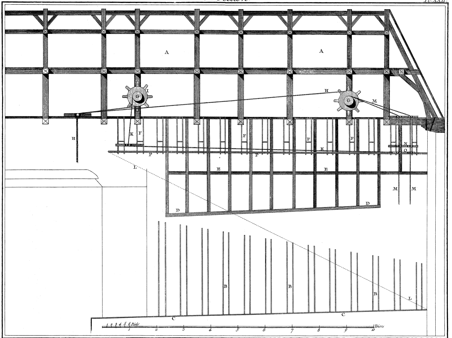
Machines de Théâtres, Élévation en Coupe sur la longueur de la Charpente du Comble et des Chemins de face avec les Corridors et Treuils pour le service des Machines, et Élévation des Châssis du Théâtre.
