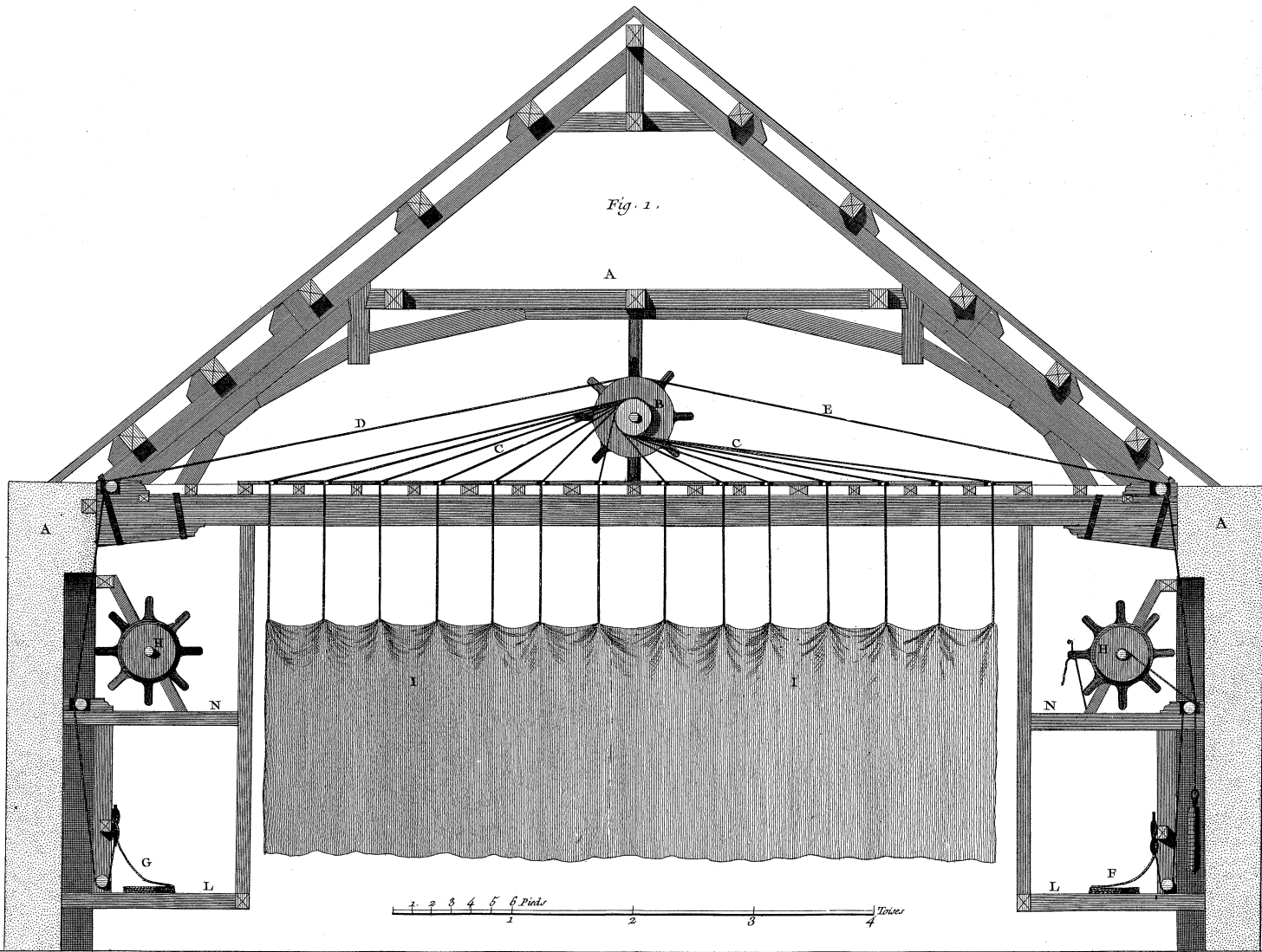
Machines de Théâtres , Élévation en Coupe de la Charpente du Comble, avec les Corridors et les Treuils pour le Service et la manœuvre du Rideau.
